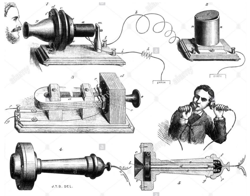
Diagramme du système téléphonique de Bell en 1877
